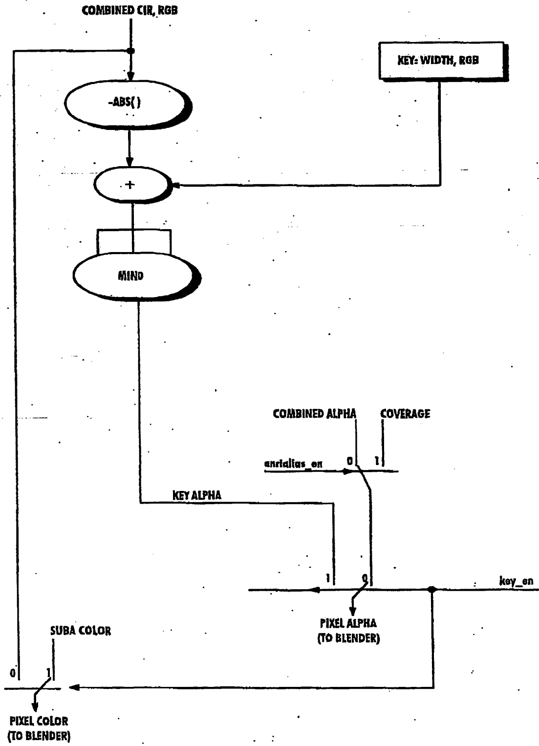
Fig. 29 ALPHA FIXUP
